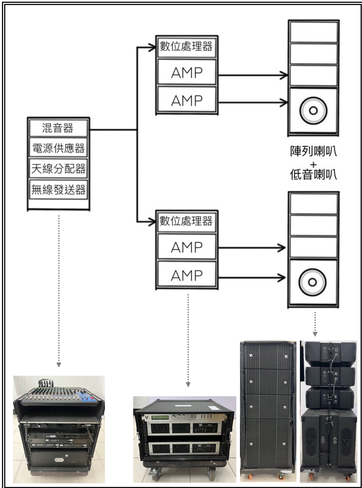
音響系統圖
