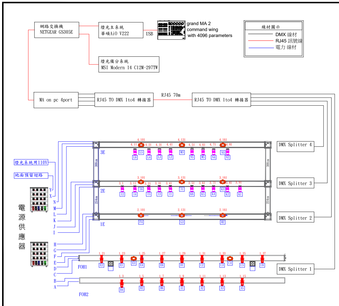
燈光系統圖
